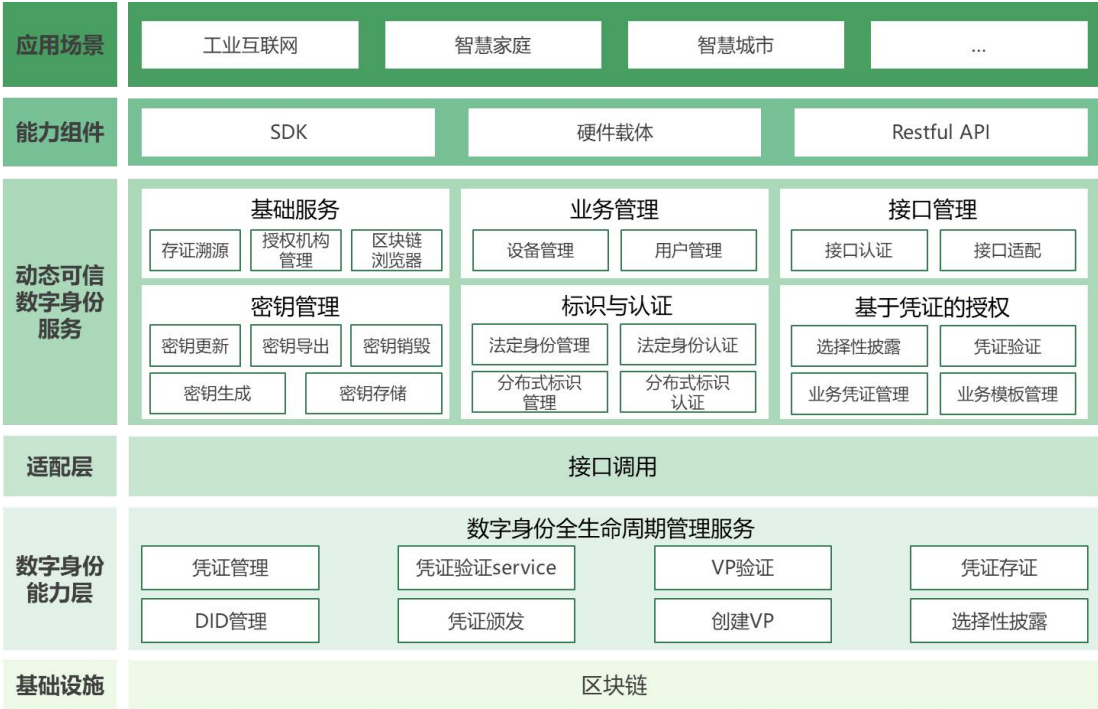
图 4-6 动态可信数字身份平台
