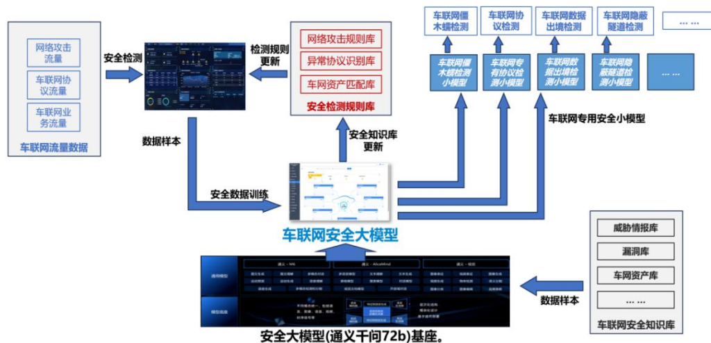
图 2-10 车联网安全大模型，形成安全资产、安全流程双闭环能力
