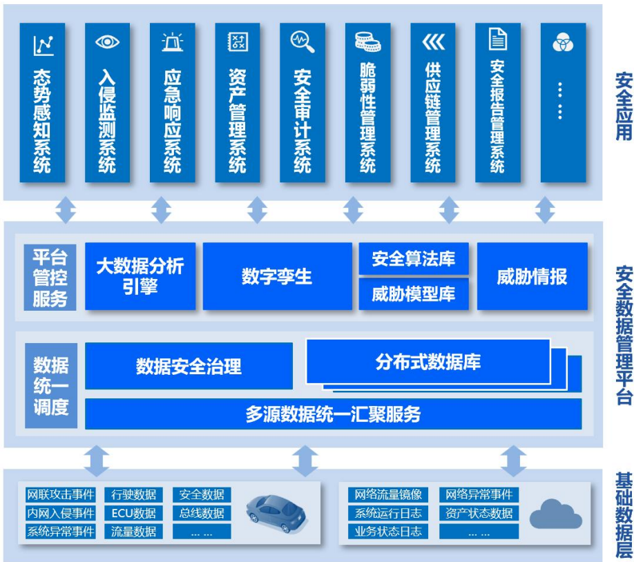
图 2-9 车联网综合安全运营的技术架构
