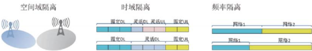
图 3-12 无线隔离
