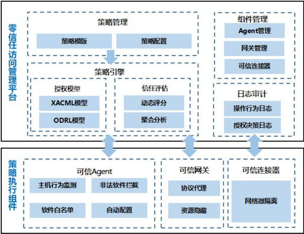
图 4-7 零信任访问管理系统
